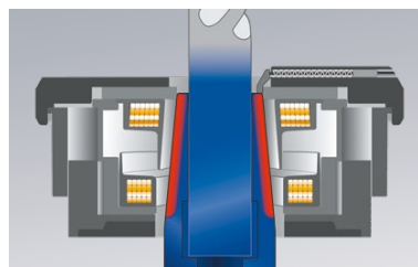
Großes Werkzeug/Big tool
