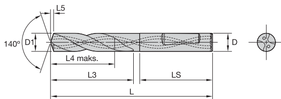
Szczegóły na temat długości L, L3 i L4 maks. znajdują się na rozkładanej stronie w tabeli wymiarów.
