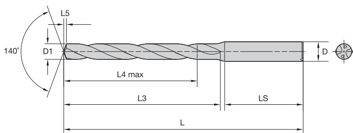
Szczegóły na temat długości L, L3 i L4 maks. znajdują się na rozkładanej stronie w tabeli wymiarów.
