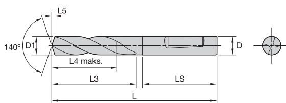
Szczegóły na temat długości L, L3 i L4 maks. znajdują się na rozkładanej stronie w tabeli wymiarów.
